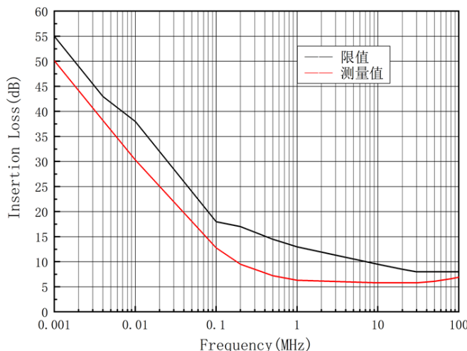
BCIP7637-3 电流注入钳插入损耗曲线
