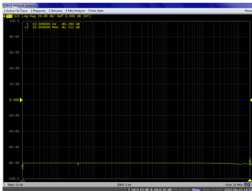
CM 0220M 宽带电流监测钳 s21 曲线*
