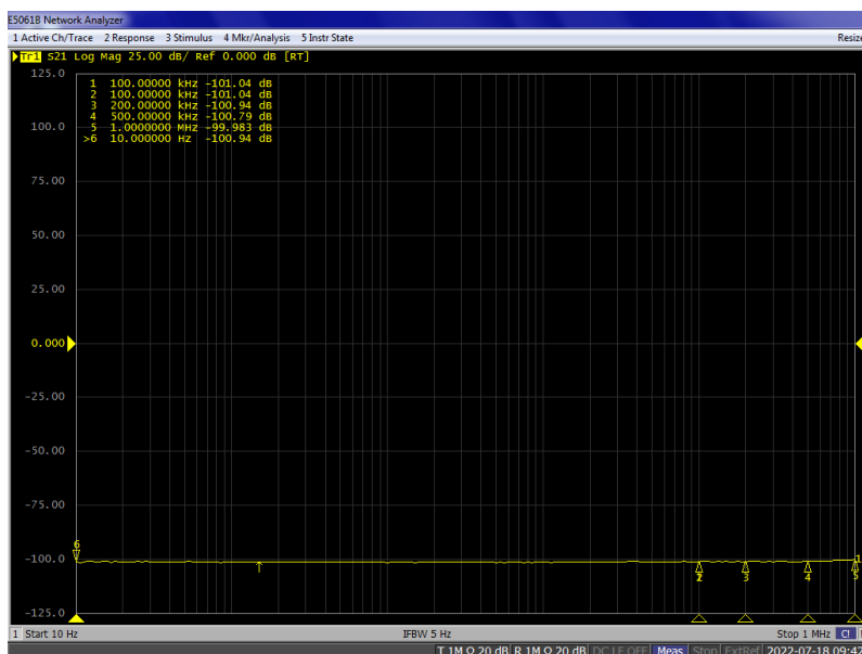
CM 0301M 宽带电流监测钳 s21 曲线*
