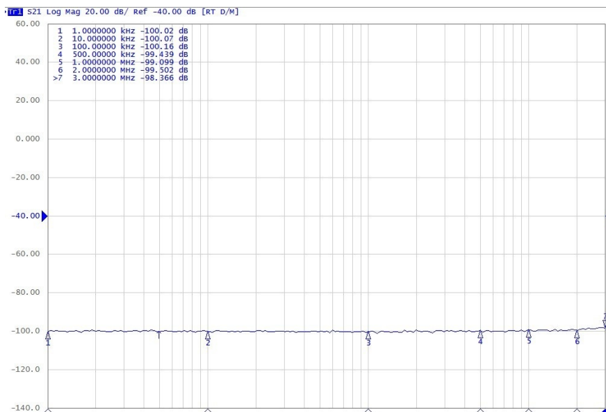
CM 0302M 宽带电流监测钳 s21 曲线*
