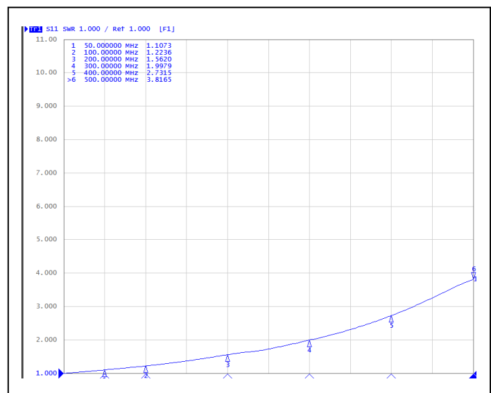
WCMCF 500 宽带电流监测钳校准夹具电压驻波比曲线
