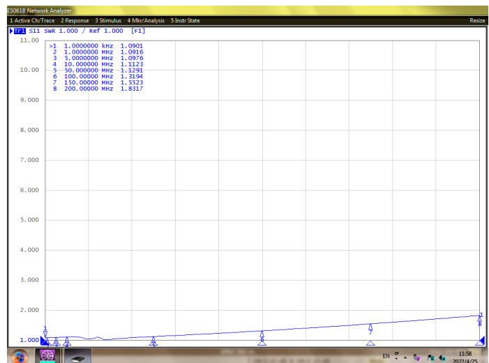
BCICF-200 电流耦合钳校准夹具电压驻波比曲线
