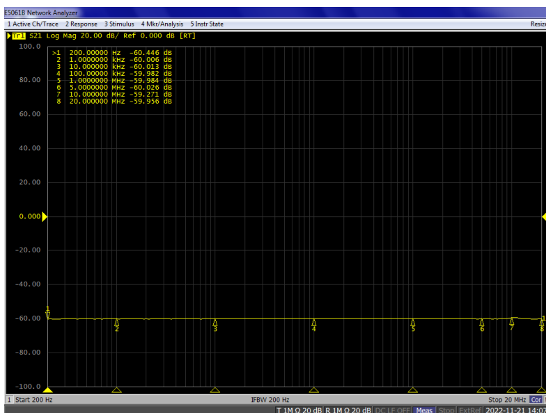
CM 0120M 宽带电流监测钳 s21 曲线*
